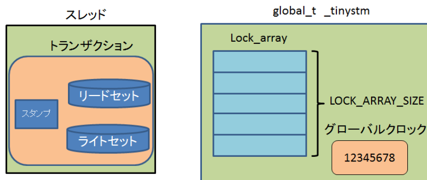
図 4.2: TinySTM の概要図
